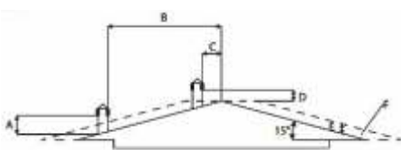
Slika 4. Krov s 15° nagiba
